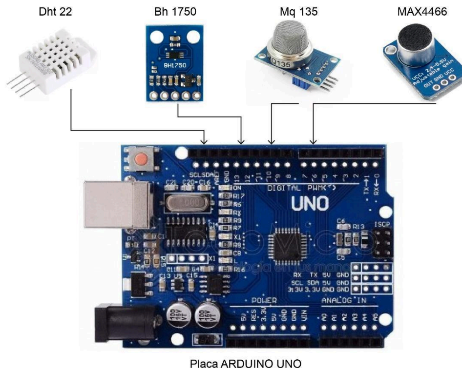
Figura 1. Estructura del hardware del sensor de IEQ.
