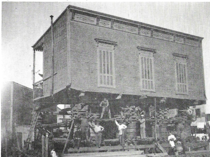
Figura 3: Rellenos, gatos y molinetes contra la inundación
